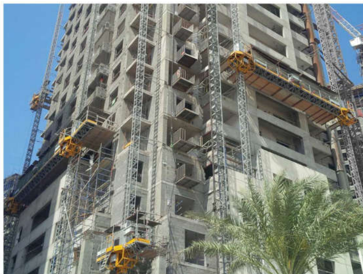
Mast climbing work platform Piattaforma di lavoro ELSA P40
